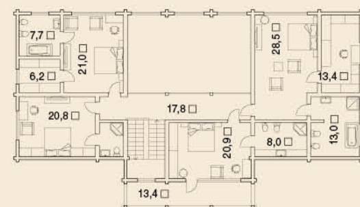
План 2 этажа
