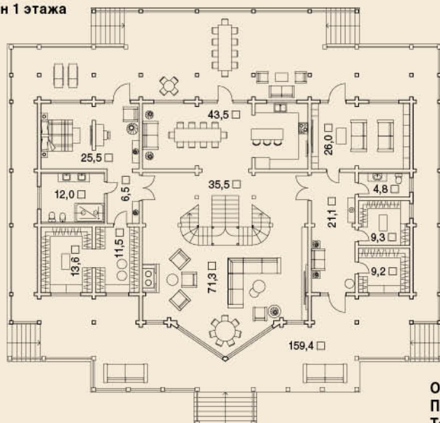
План 1 этажа
